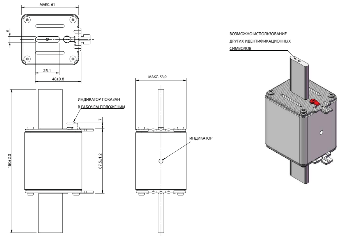
NH размер 2
