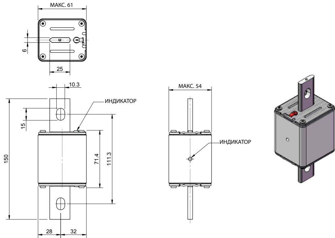
НН размер 2
