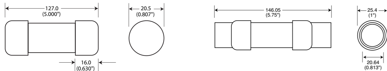
20 × 127 мм 5–30 А
