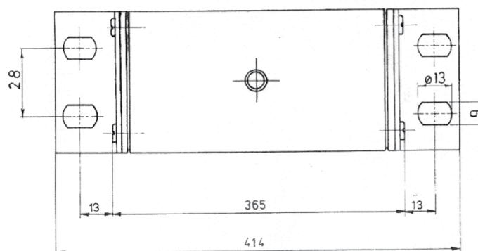
Тип 2SKN/394
