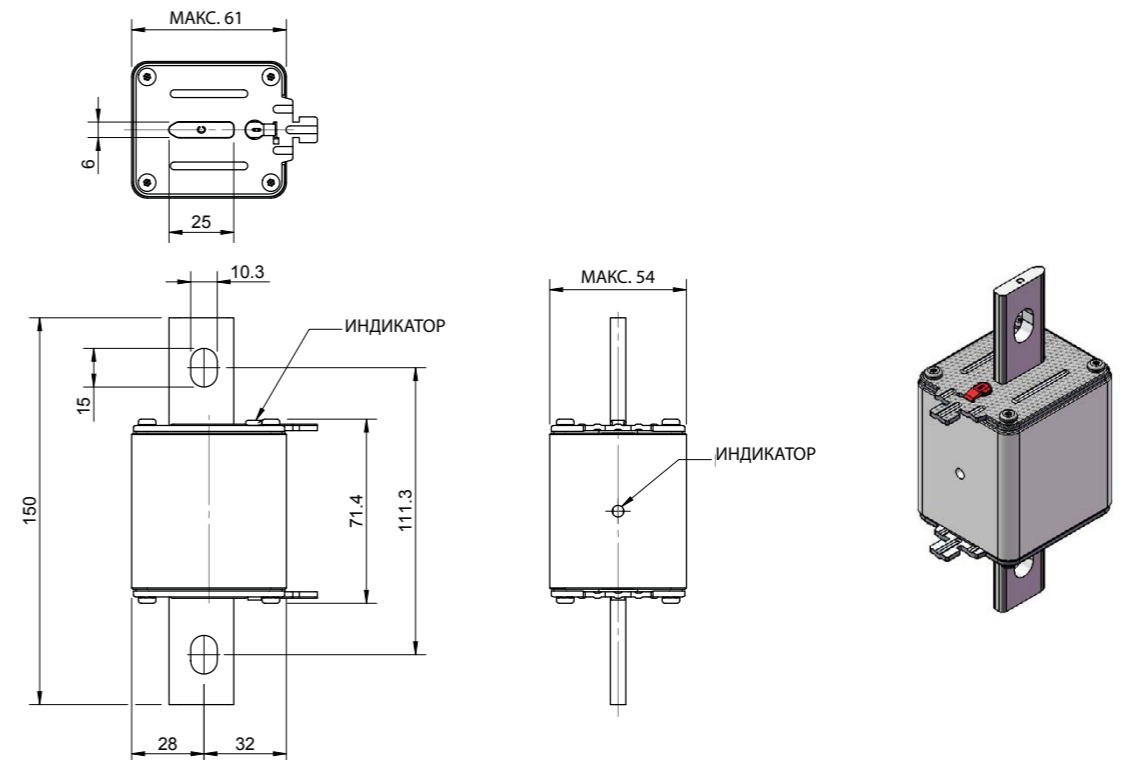
НН размер 2
