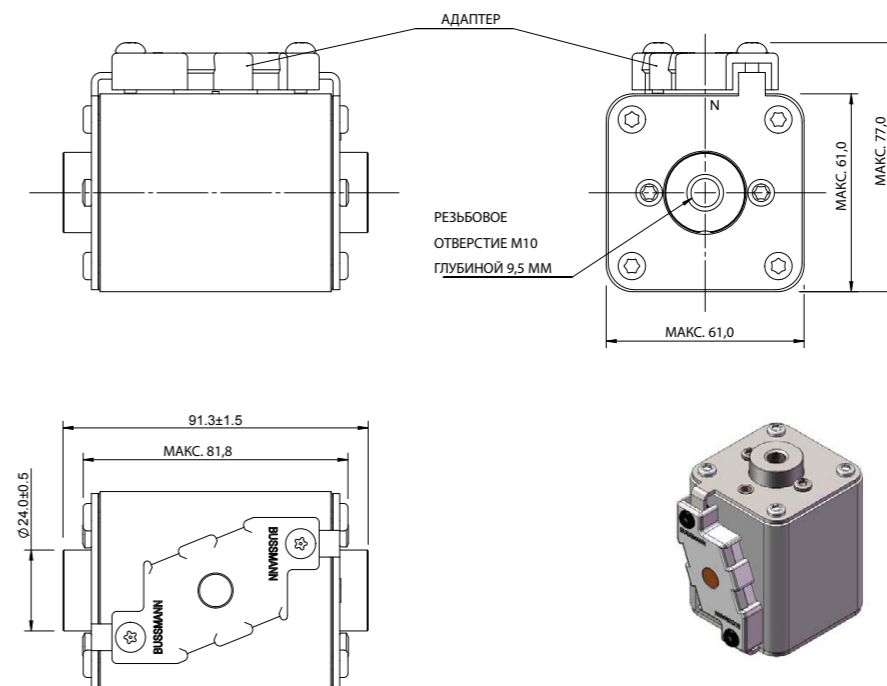
НН размер 2
