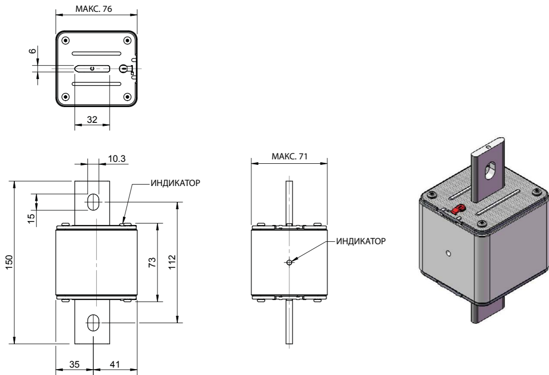
НН размер 3
