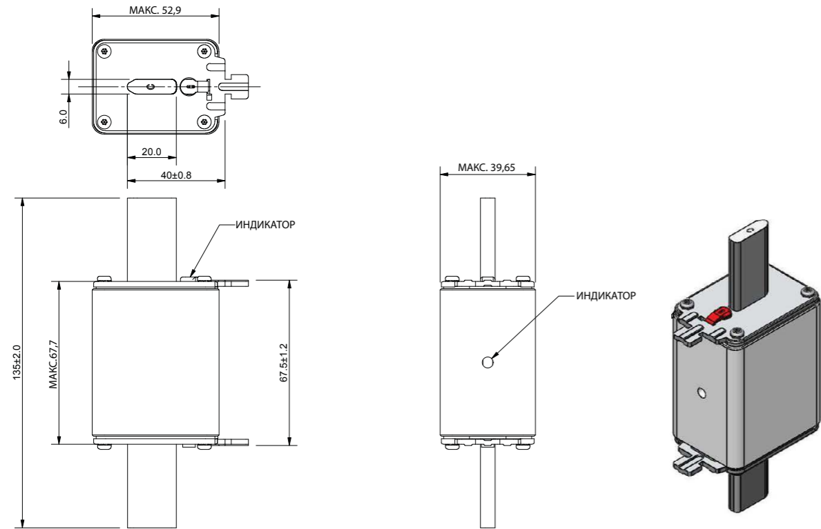
NH размер 1
