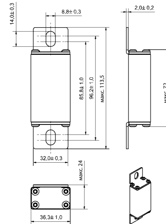
Размер 000
