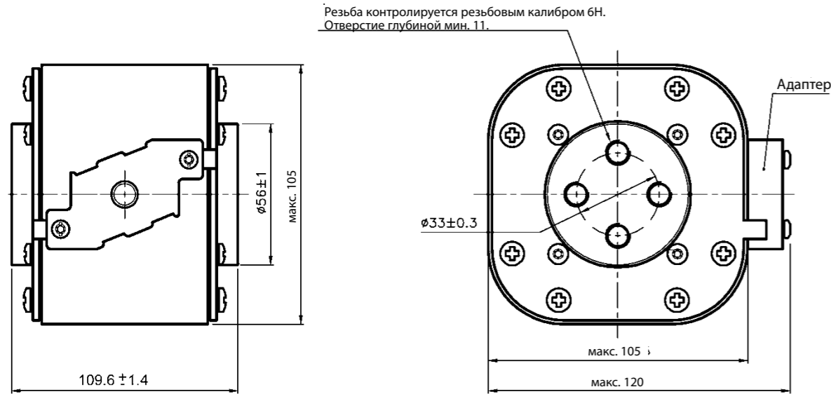
Тип 4BKN/105
