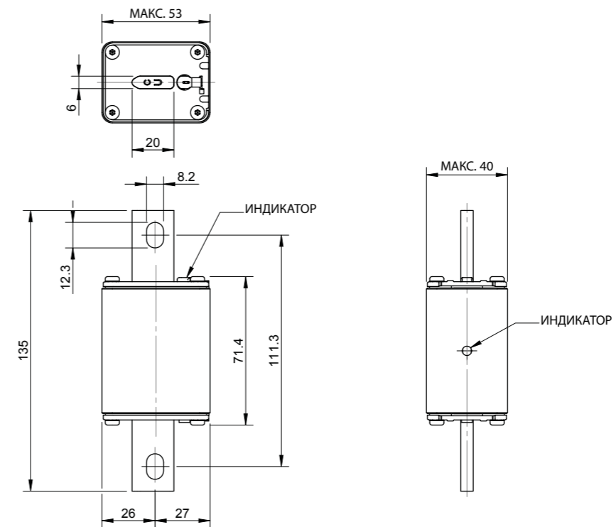
NH размер 1
