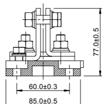
РАЗРЕЗ A-A
