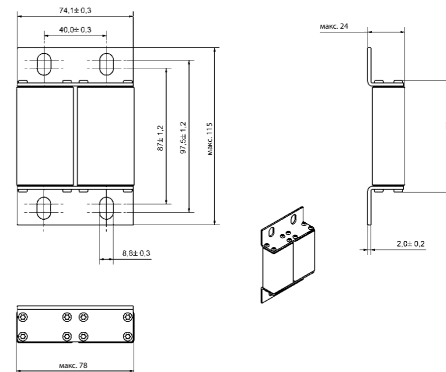
Размер 230
