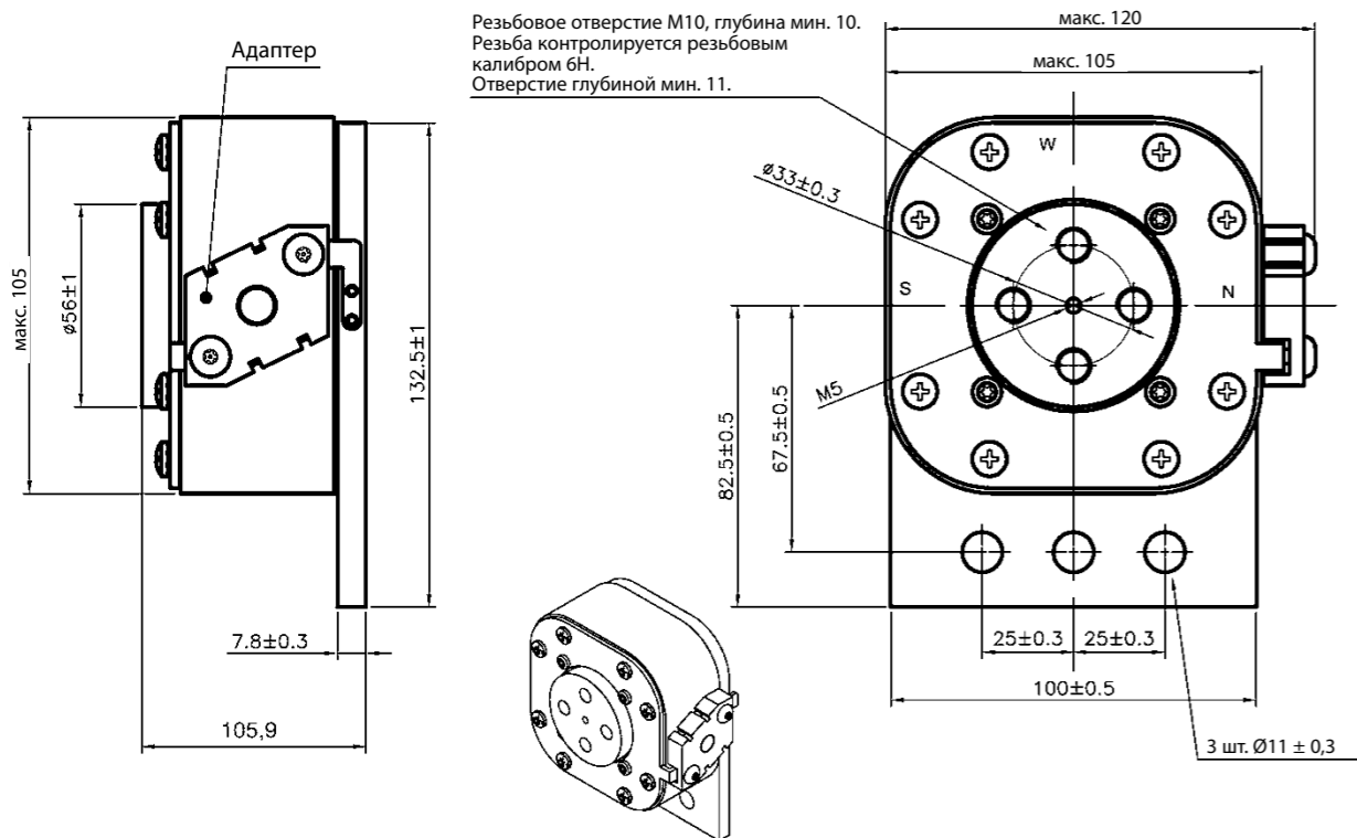
Тип 4SBKN/105
