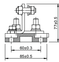
РАЗРЕЗ A-A
