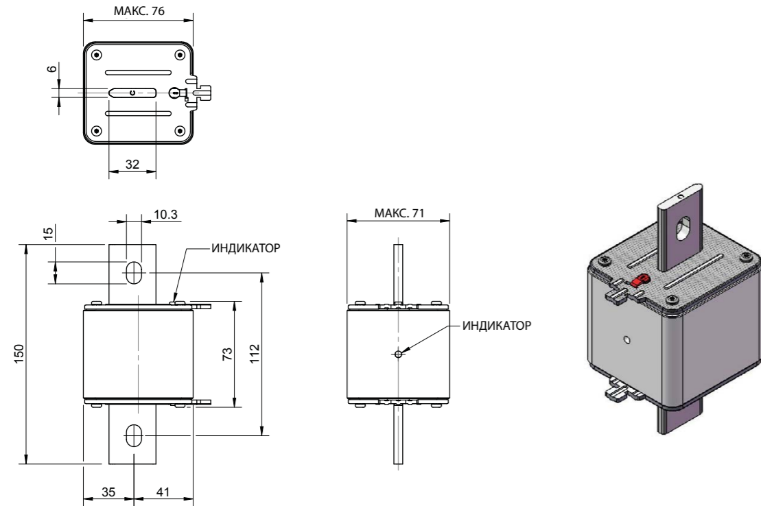
НН размер 3
