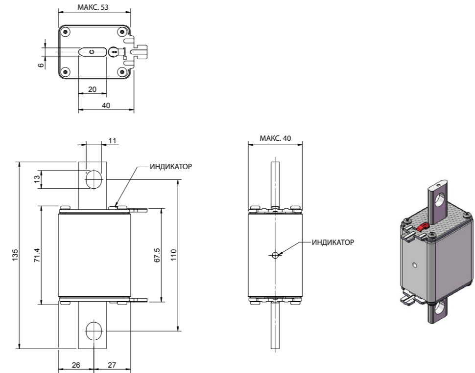
НН размер 1
