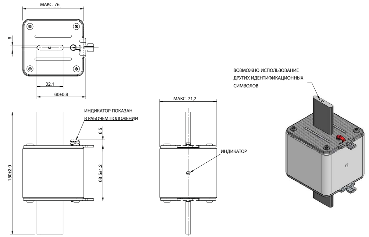
NH размер 3
